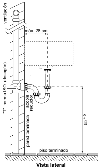
Vista lateral
